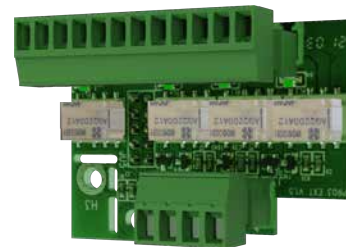
PR1 - Reläkort till Omnis PSU 5A-10A
